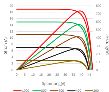
Strom-Spannungs- und Leistungs-Spannungs-Diagramme (710W)
